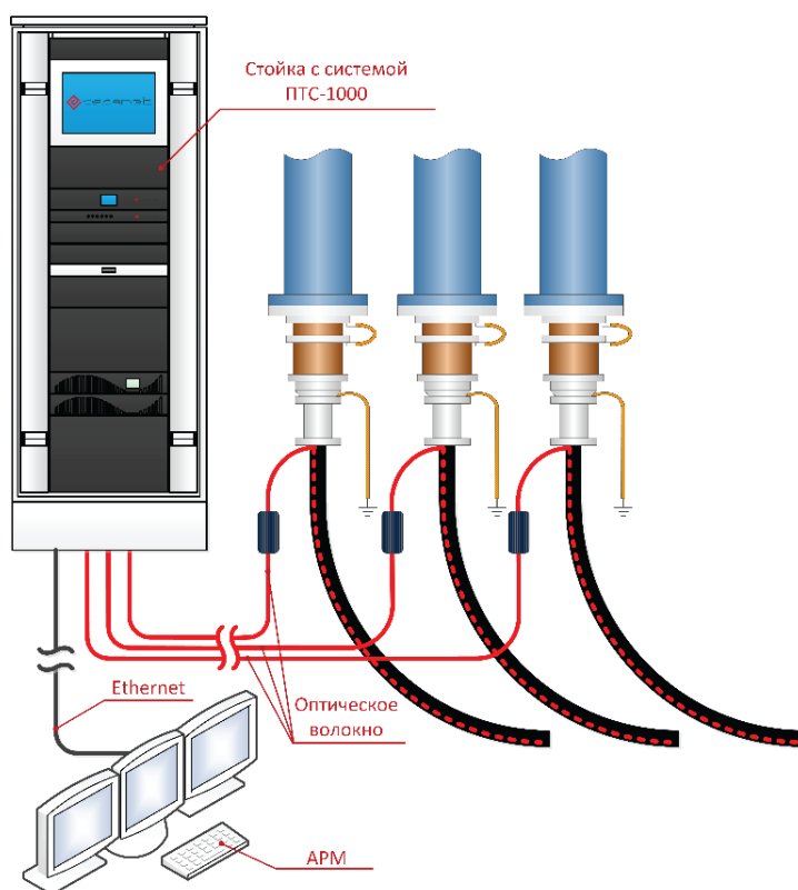
Схема подключения основных компонентов системы ПТС-1000.
